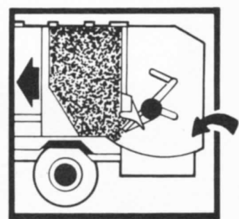
SURCOMPRESSION DES ORDURES MENAGERES CONTRE UNE PAROI MOBILE AVEC UN FORT COEFFICIENT DE TASSEMENT.
